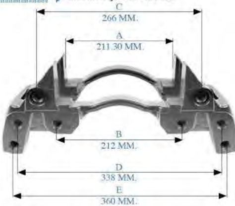
KP 320 0277 >> BALATA TAŞIYICI / CARRIER
