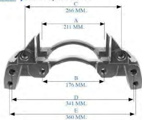
KP 320 0278 >> BALATA TAŞIYICI / CARRIER
